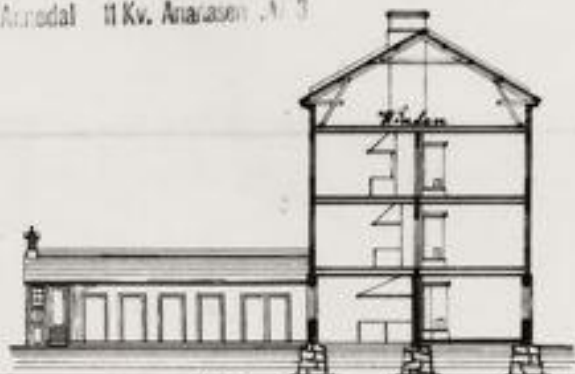
sektion A-B
